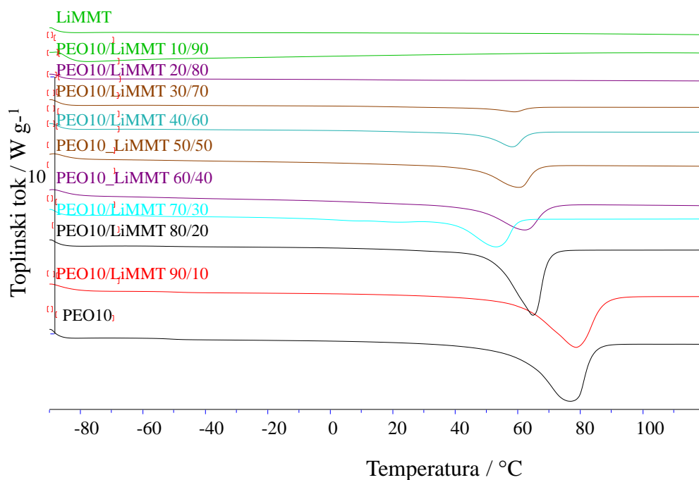
Slika 68. Normalizirane DSC krivulje drugog ciklusa zagrijavanja PEO10, LiMMT i nanokompozita PEO10/LiMMT
