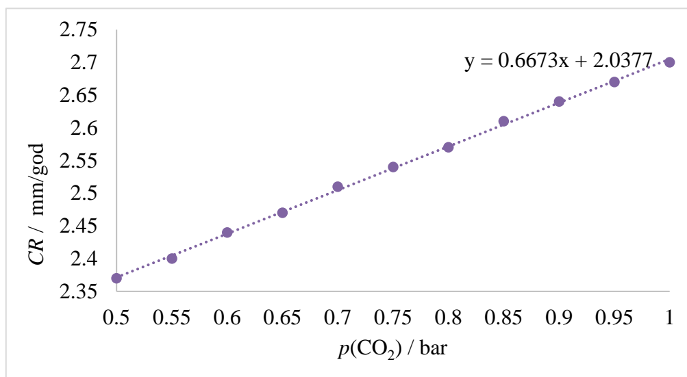
Slika 24. Prikaz ovisnosti brzine korozije niskougličnog čelika o promjeni parcijalnog tlaka CO 2 od 0,5 bar do 1 bar pri zadanim uvjetima ( T = 20 \text{ }^\circ\text{C} , p(\text{ukupni}) = 2 \times p(\text{CO}_2) , d_u = 0,1 \text{ m} , \text{pH} = 4 , v = 2 \text{ m/s} , c(\text{Fe}^{2+}) = 100 \text{ ppm} )
