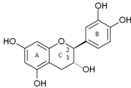
Slika 3. Struktura katehina
