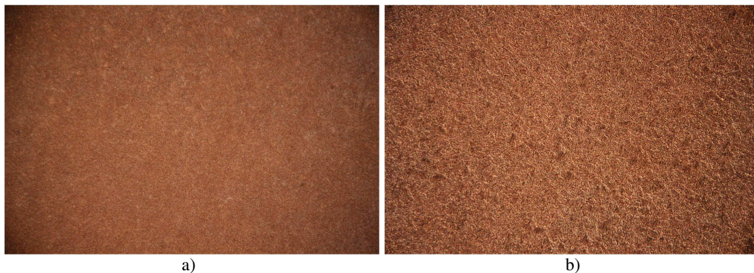
Slika 22. Površina Cu elektrode nakon potenciodinamičkog polarizacijskog mjerenja u 0,5 \text{ mol dm}^{-3} NaCl otopini uz uvećanje a) 100\times i b) 200\times
