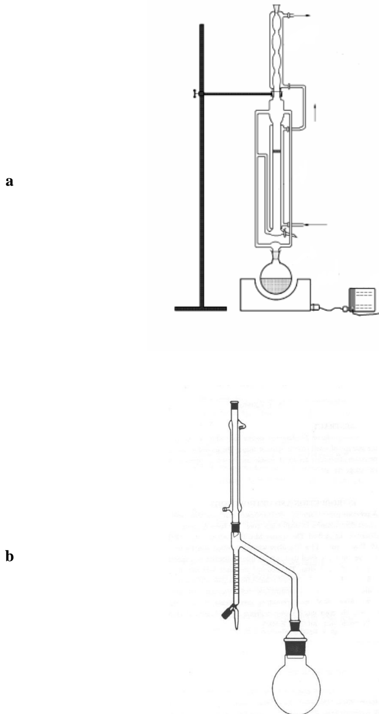
Slika 7. Različite aparature za hidrodestilaciju alga: a) modificirana aparatura po Clevengeru (preuzeto i prilagođeno iz M. Zekić) 32 , b) modificirana Dean-Stark aparatura (preuzeto i prilagođeno iz N. T. Faithfull i V. Gressler i sur.) 29,33
