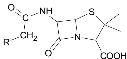
Slika 13. Monosupstituirani metilpenicilin
