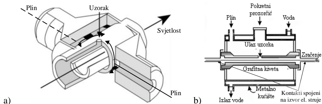
Slika 11. a) Grafitna kiveta 24 ; b) Prikaz grafitne kivete u peći 13
