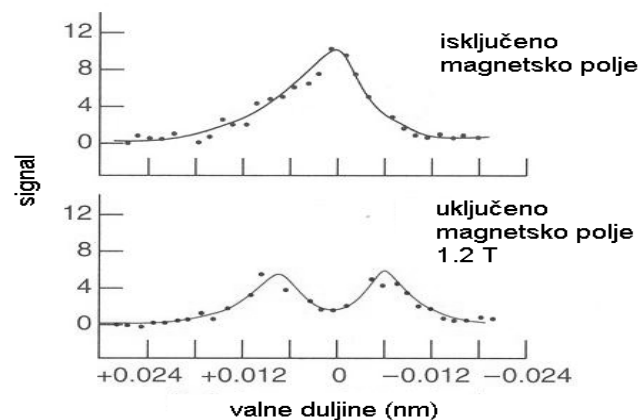
Slika 14. Zeemanov efekt 29
