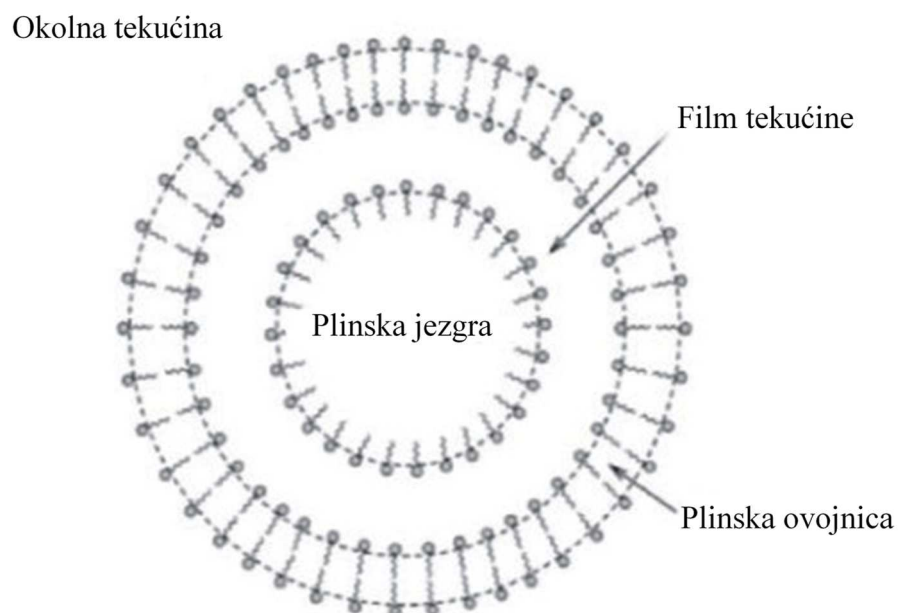
Slika 1.6. Struktura mikromjehurića. 12
