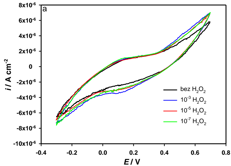
Slika 20a. Utjecaj dodatka H_2O_2 na CV pri pH 5. Elektroda MWCNT-MnO 2 -10
