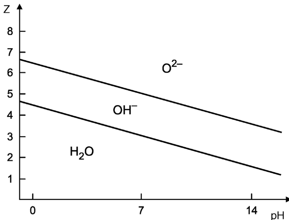
Slika 12 Valencija (Z) - pH dijagram koji ukazuje na područja akva, hidroksidna i oksidna vrsta 5
