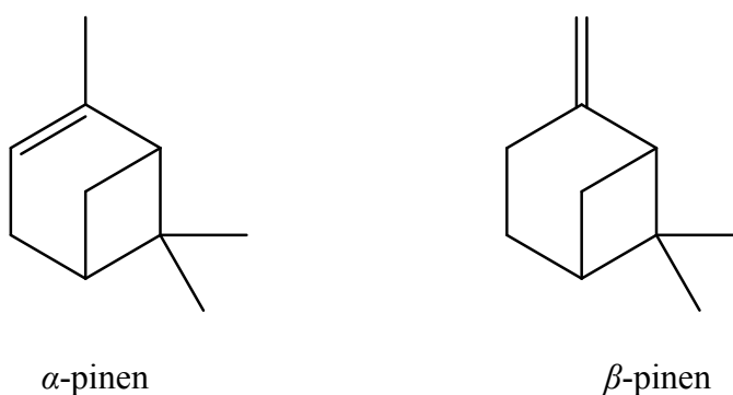
Slika 7. Strukture \alpha - i \beta -pinena 10
