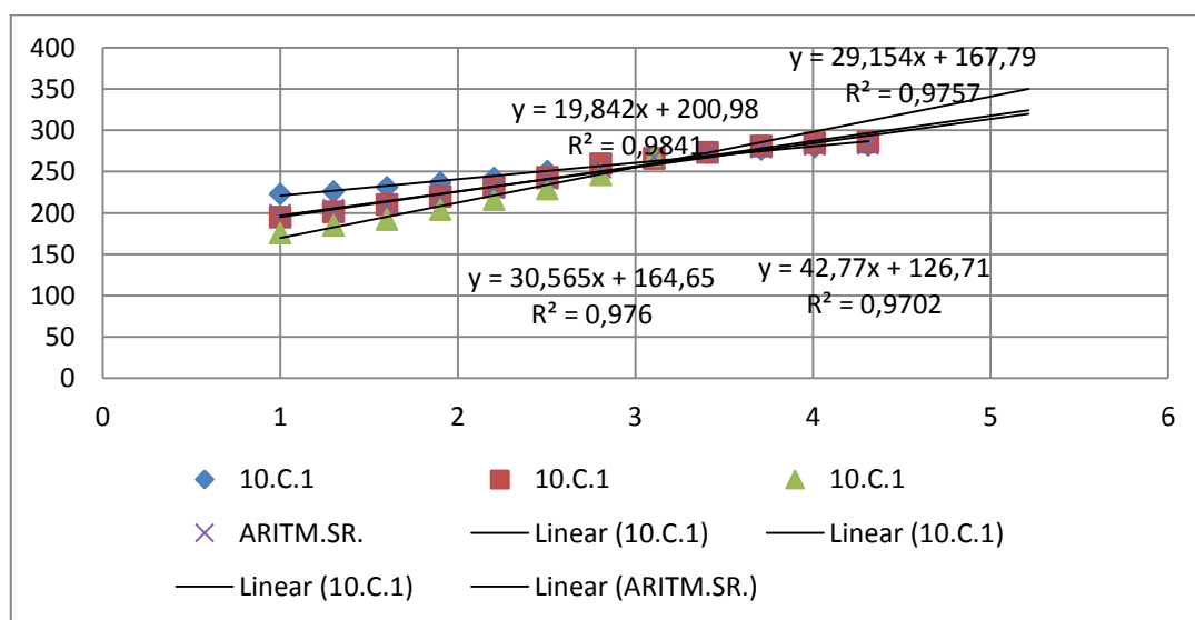
Slika 16. Prikaz ispitivanja odziva elektrode na Fe 2+ ione
