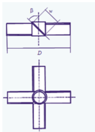
Slika 16. PBT miješalo
