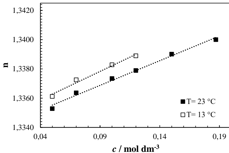
Slika 28. Baždarni pravci ovisnosti refraktivnog indeksa o koncentraciji otopine boraksa pri T = 23 i 13 °C
