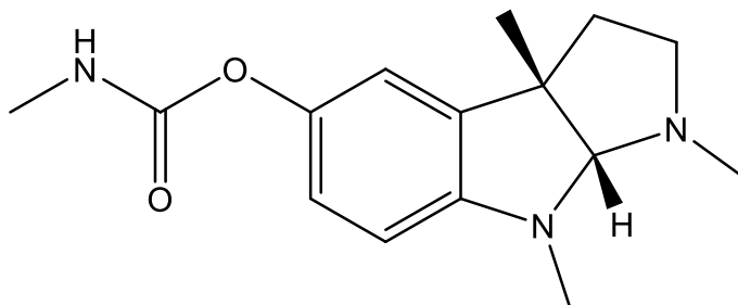
Slika 8. Struktura fizostigmina
