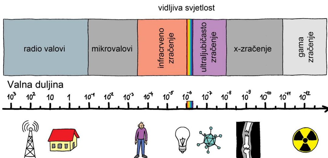
Slika 1.11. Elektromagnetski spektar 23
