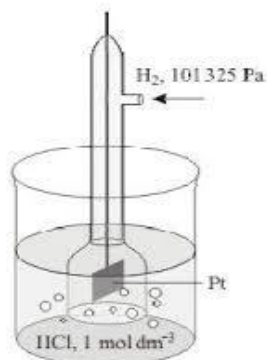
Slika 3. Standardna vodikova elektroda 6
