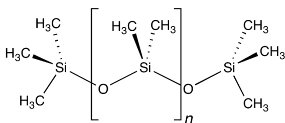
Slika 9: Prikaz dimetilpolisiloksana
