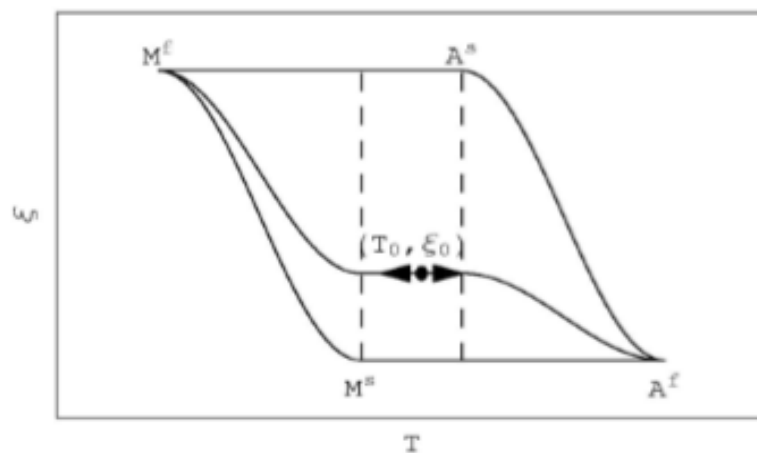
Slika 3. Prikaz temperaturne martenzitne transformacije i temperaturne histereze 7
