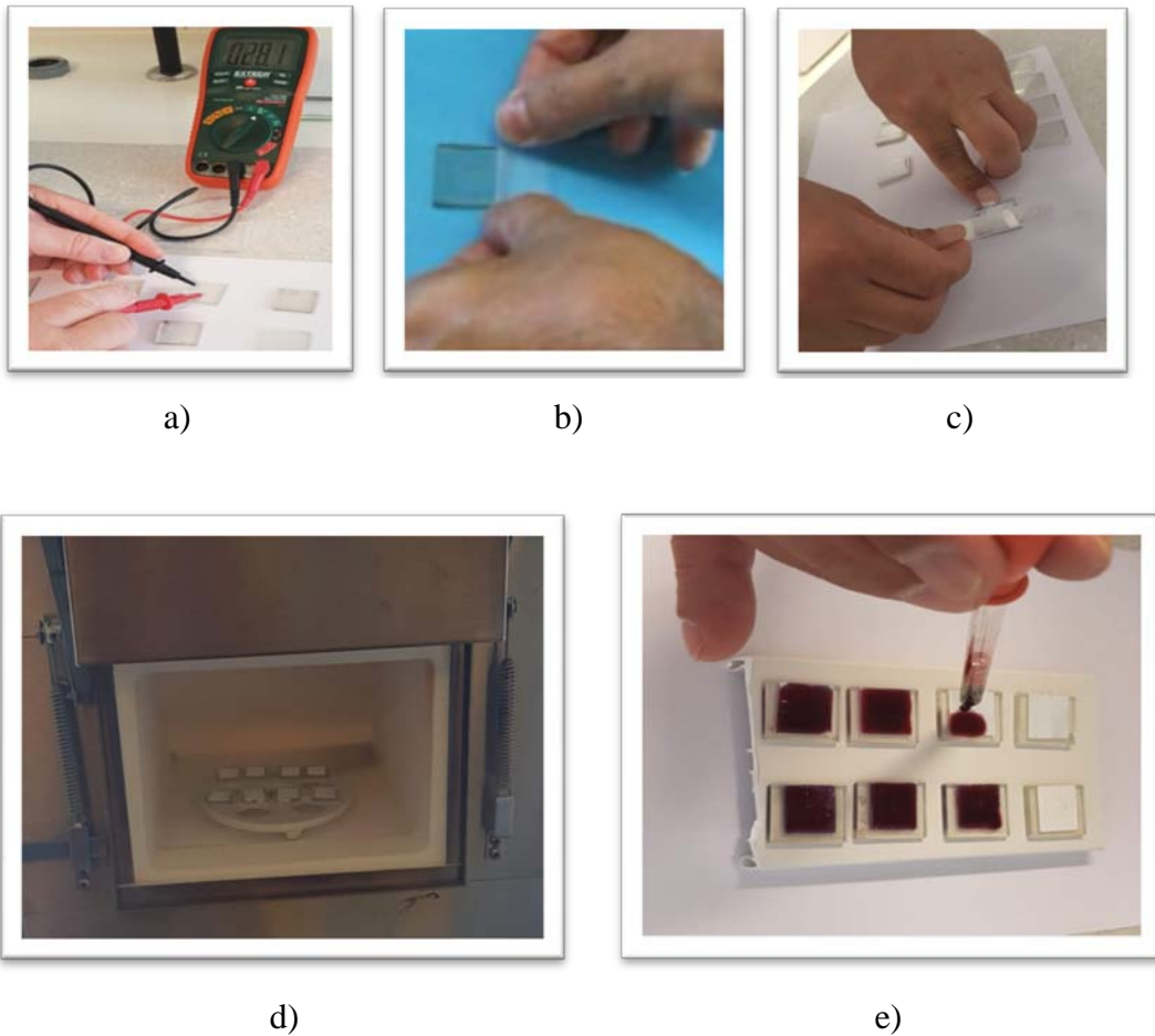
Slika 14. Postupak izrade pločice s poroznim slojem nanokristaličnog TiO 2
