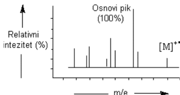
Slika 13. Spektar masa. 4
