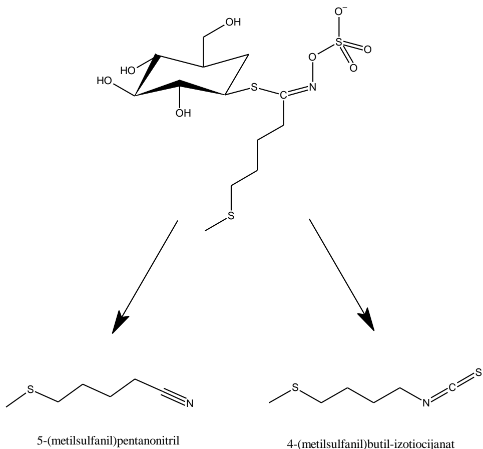
Slika 39. Razgradnja glucoerucina.
