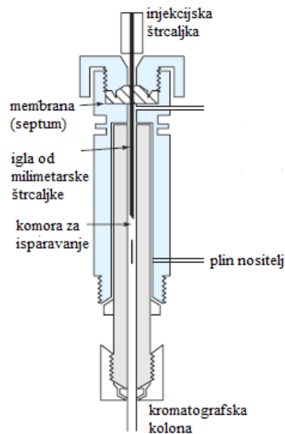
Slika 8 Injektor za ubacivanje uzorka u plinski kromatograf (20)
