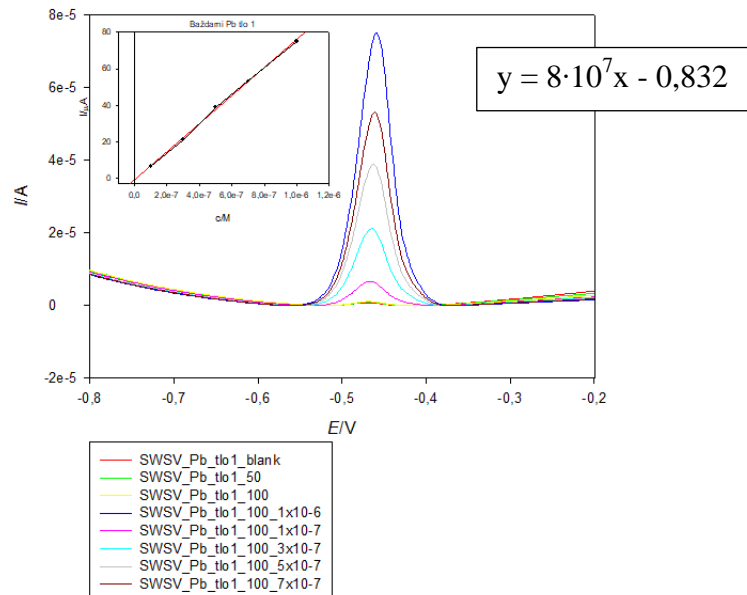
Slika 32. Normalizirani voltamogrami anodne „stripping“ voltametrije za određivanje Pb^{2+} u uzorku TLO 1 (metodom standardnog dodatka) na GCE-Hg. Parametri: vrijeme akumulacije: 60 s, vrijeme stabilizacije: 30 s, amplituda: 0,025 V, broj ciklusa: 3, frekvencija: 10 \text{ s}^{-1} , početni potencijal: -1 V, krajnji potencijal: +0,25 V, step potencijal: 0,00195 V. Umetnut: krivulja umjeravanja ovisnosti gustoće struje o koncentraciji Pb^{2+}
