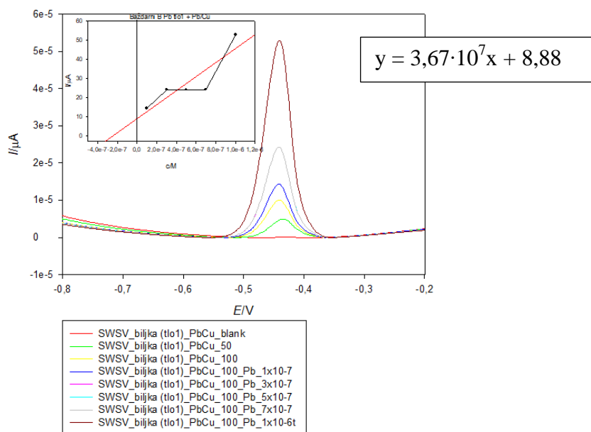
Slika 40. Normalizirani voltamogrami anodne „stripping“ voltometrije za određivanje Pb 2+ u uzorku biljke TLO 1 (metodom standardnog dodatka) zalijevanim s Pb/Cu na GCE-Hg. Parametri: vrijeme akumulacije: 60 s, vrijeme stabilizacije: 30 s, amplituda: 0,025 V, broj ciklusa: 3, frekvencija: 10 s -1 , početni potencijal: -1V, krajnji potencijal: +0,25 V, step potencijal: 0,00195 V. Umetnut: krivulja umjeravanja ovisnosti gustoće struje o koncentraciji Pb 2+
