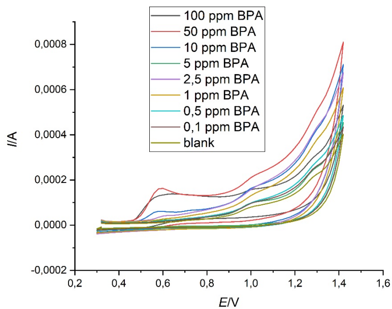
Slika 19a - ciklički voltamogrami na CPE u ovisnosti o koncentraciji BPA pri koncentraciji imobilizirane DNA 10 mgL -1
