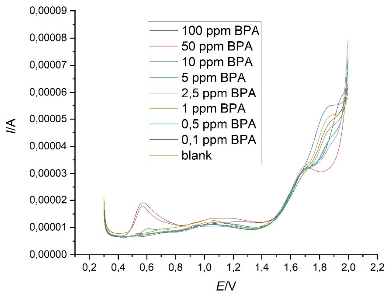
Slika 24e - DP voltamogrami na BDDE u ovisnosti o koncentraciji BPA pri koncentraciji DNA 500 mgL -1
