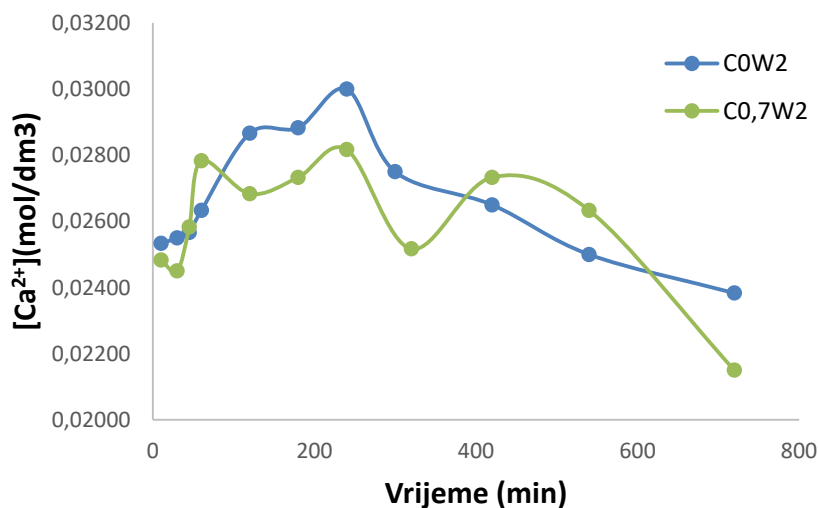
Slika 26. Koncentracija \text{Ca}^{2+} iona za cement oznake C0W2 i C0,7W2
