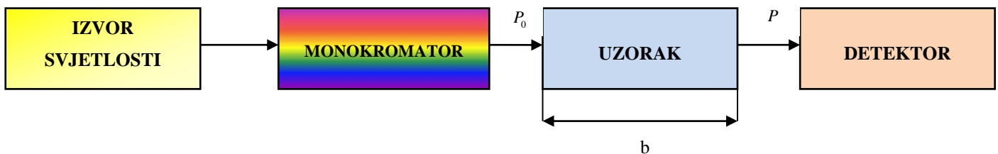
Slika 2-3 Shematski dijagram jednosnognog spektrometrijskog eksperimenta
