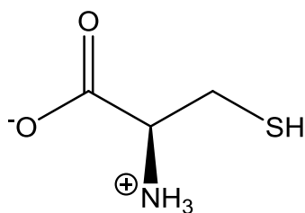
Slika 1.3. Struktura L-α-cisteina ( zwitter ion)
