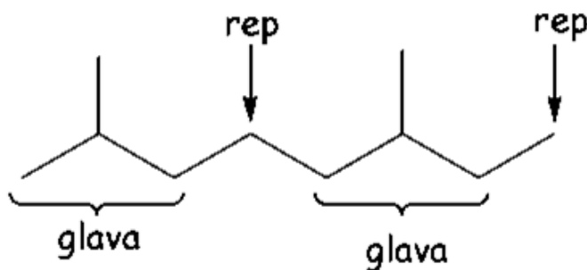
Slika 1.4. Izoprensko pravilo
