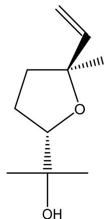
trans -linalol oksid
