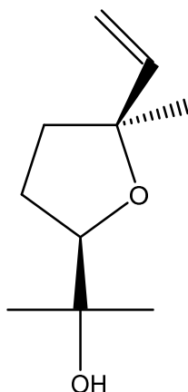
cis -linalol oksid
