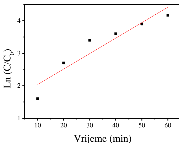
Slika 11. Promjena koncentracije MO bojila s vremenom izlaganja zračenju svjetiljke
