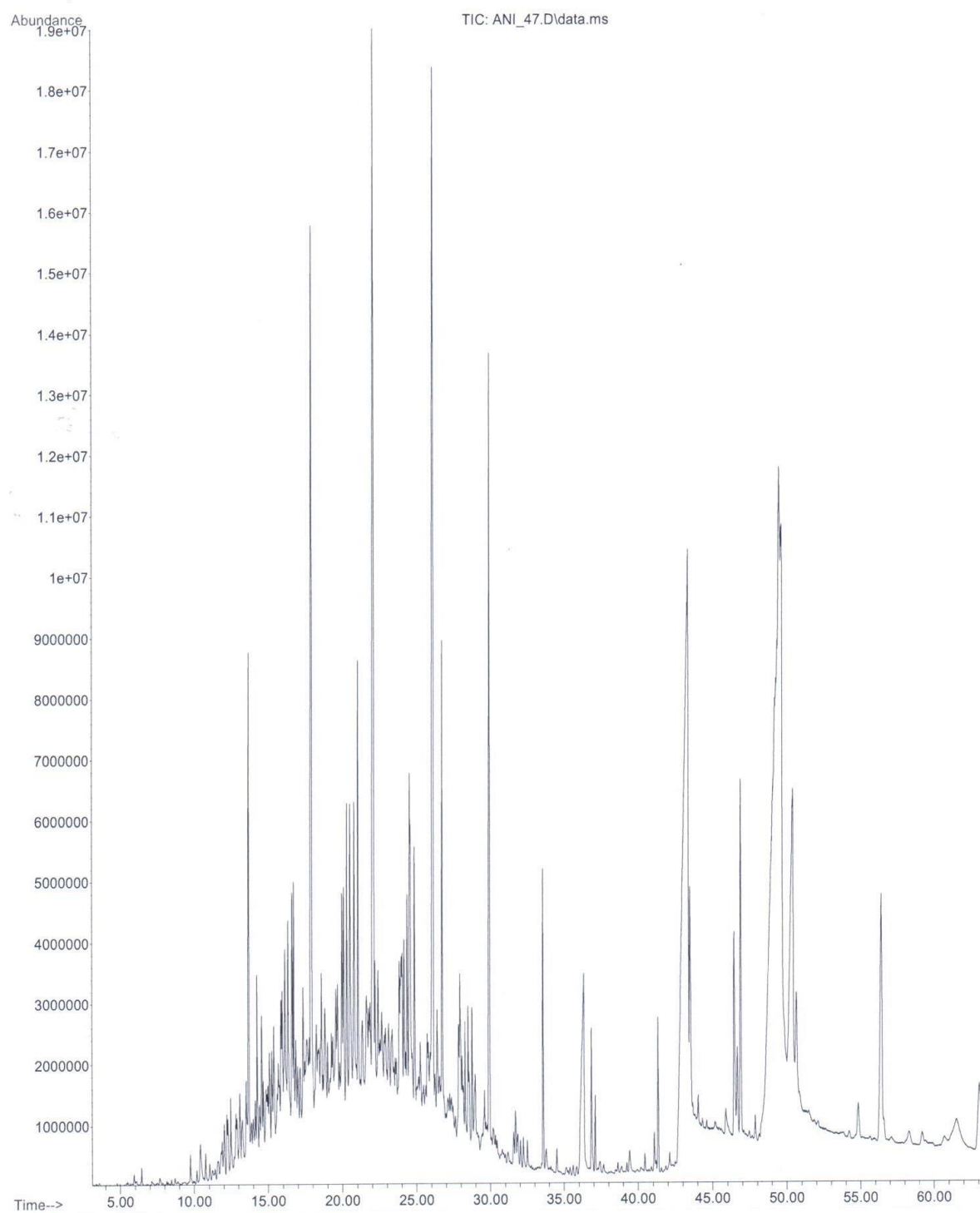
Slika 17. Kromatogram apsoluta 2
