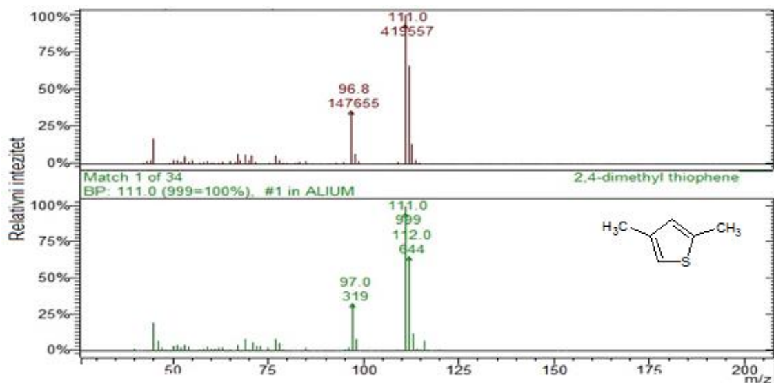
Slika 3.21. Spektar masa 2,4-dimetil tiofena
