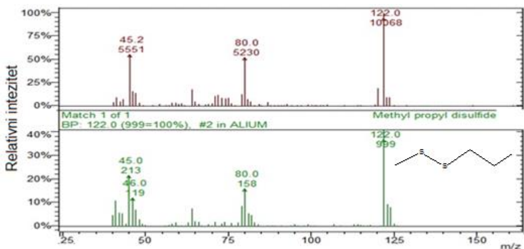
Slika 3.17. Maseni spektar metilpropil disulfida
