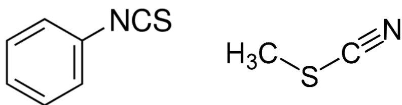
Slika 1.5. Četvrta grupa sumporovih spojeva 2
