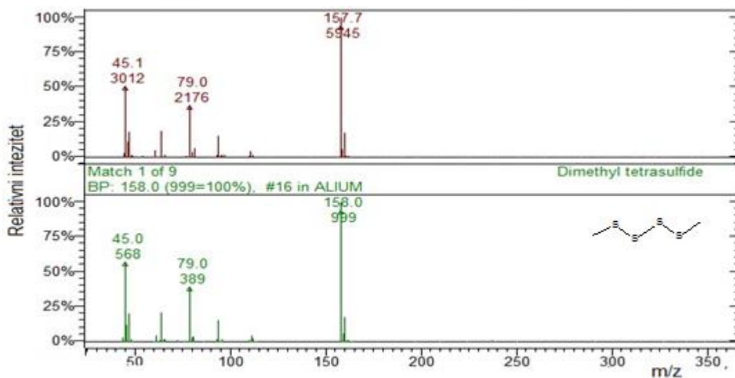
Slika 3.20. Maseni spektar dimetil tetrasulfid
