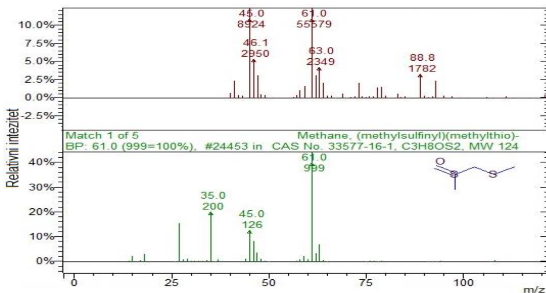
Slika 3.22. Spektar masa (metilsulfinil)(metilsulfanil)metana
