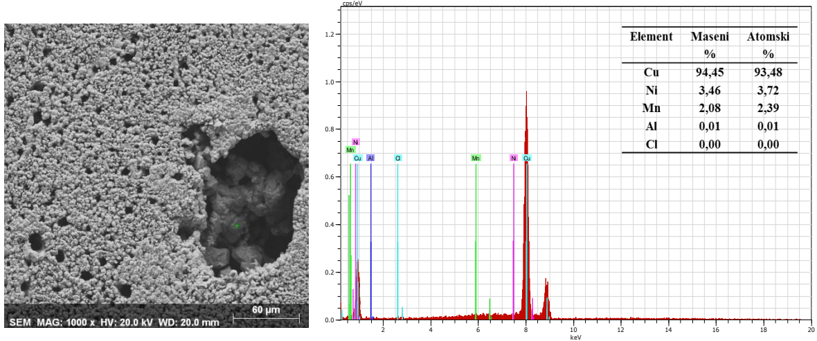
Slika 36. SEM snimke površine uzorka CuAlNiMn legure nakon polarizacijskog mjerenja u mirujućoj 0,9 % NaCl otopini ( \text{pH} = 7,4 i T = 50\text{ }^{\circ}\text{C} ) uz uvećanje 1000 puta a) i c) i pripadajuće EDS analize b) i d)
