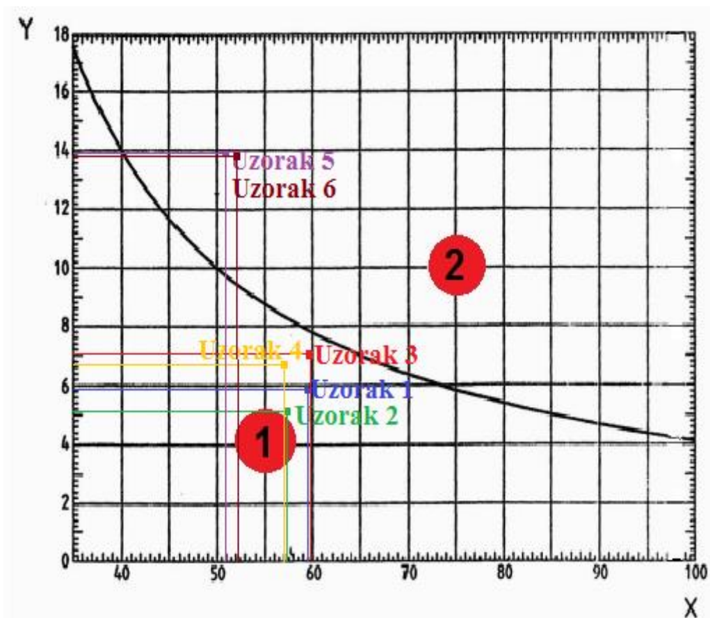
Slika 11. Dijagram izotermne topljivosti \text{Ca}(\text{OH})_2 u ovisnosti o ukupnom alkalitetu otopine iznad uzorka pucolanskog cementa gdje je:
