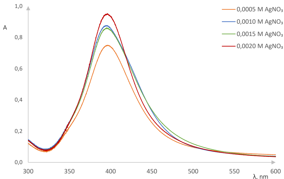
Slika 19. Apsorpcijski spektar četvrte serije otopina
