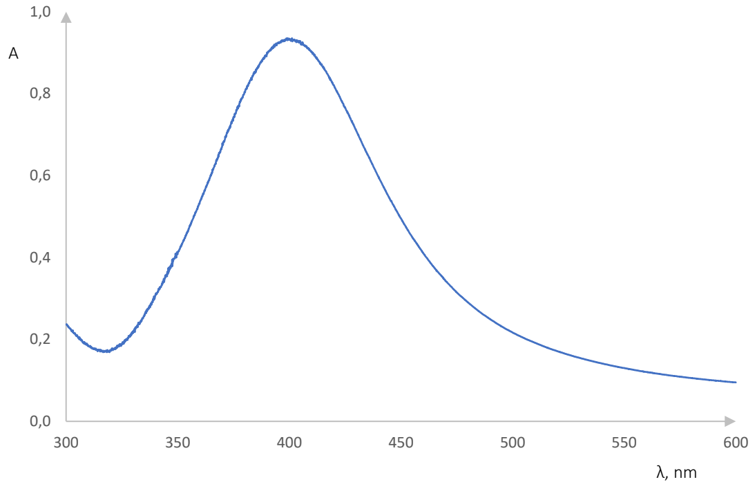
Slika 23. Apsorpcijski spektar pri koncentraciji \text{AgNO}_3 0,0005 mol/dm 3
