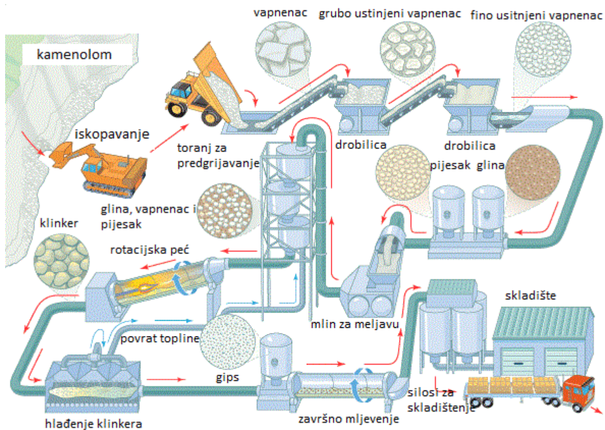
Slika 1. Shema proizvodnje portlandskog cementa [3]
