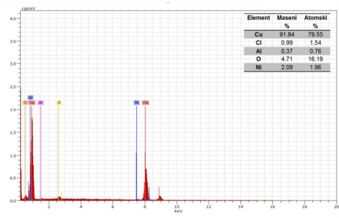
Slika 30. SEM snimka površine uzorka CuAlNi legure nakon potenciodinamičkog polarizacijskog mjerenja u 0.1 % NaCl otopini (uvećanje 2000 puta) i pripadajuća EDS analiza
