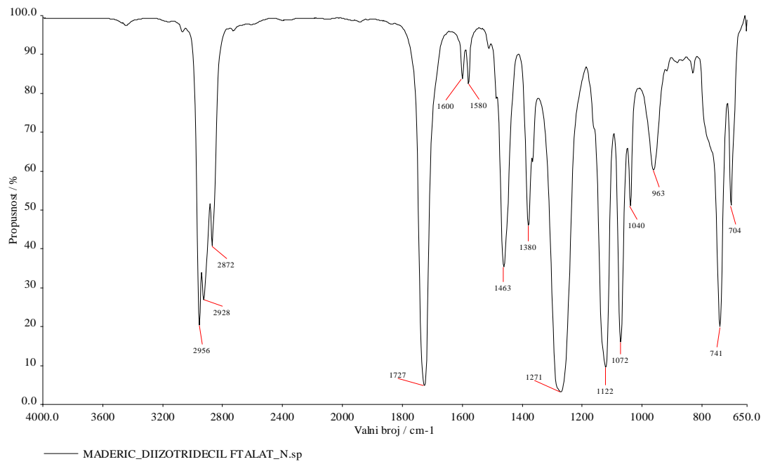
Slika 51. FT-IR spektar diizotridecil ftalata
