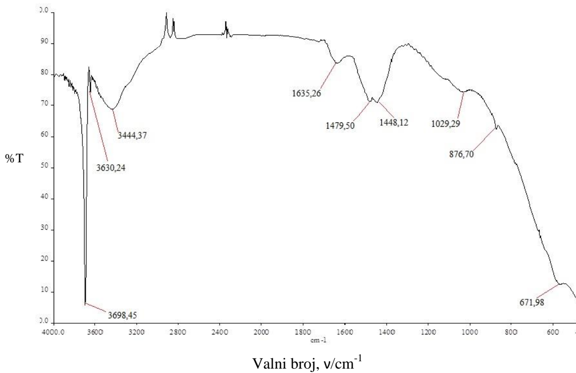
Valni broj, \nu/\text{cm}^{-1} Slika 11. FT-IR spektar nemodificiranog magnezijeva hidroksida
