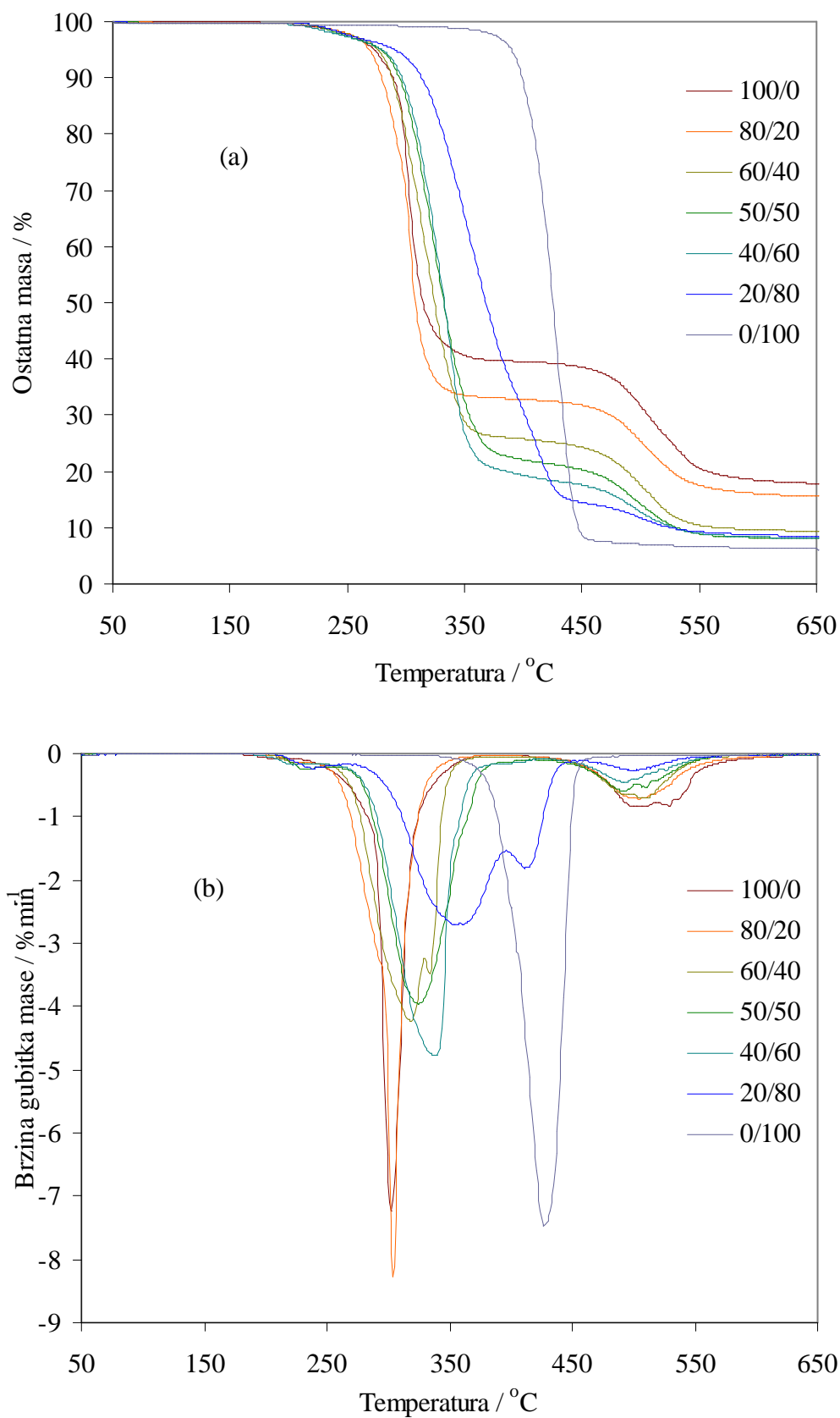
Slika 51. TG (a) i DTG (b) krivulje dinamičke TG razgradnje mješavina PVC/PEO3 različitog sastava u inertu pri brzini zagrijavanja 2,5 °Cmin -1
