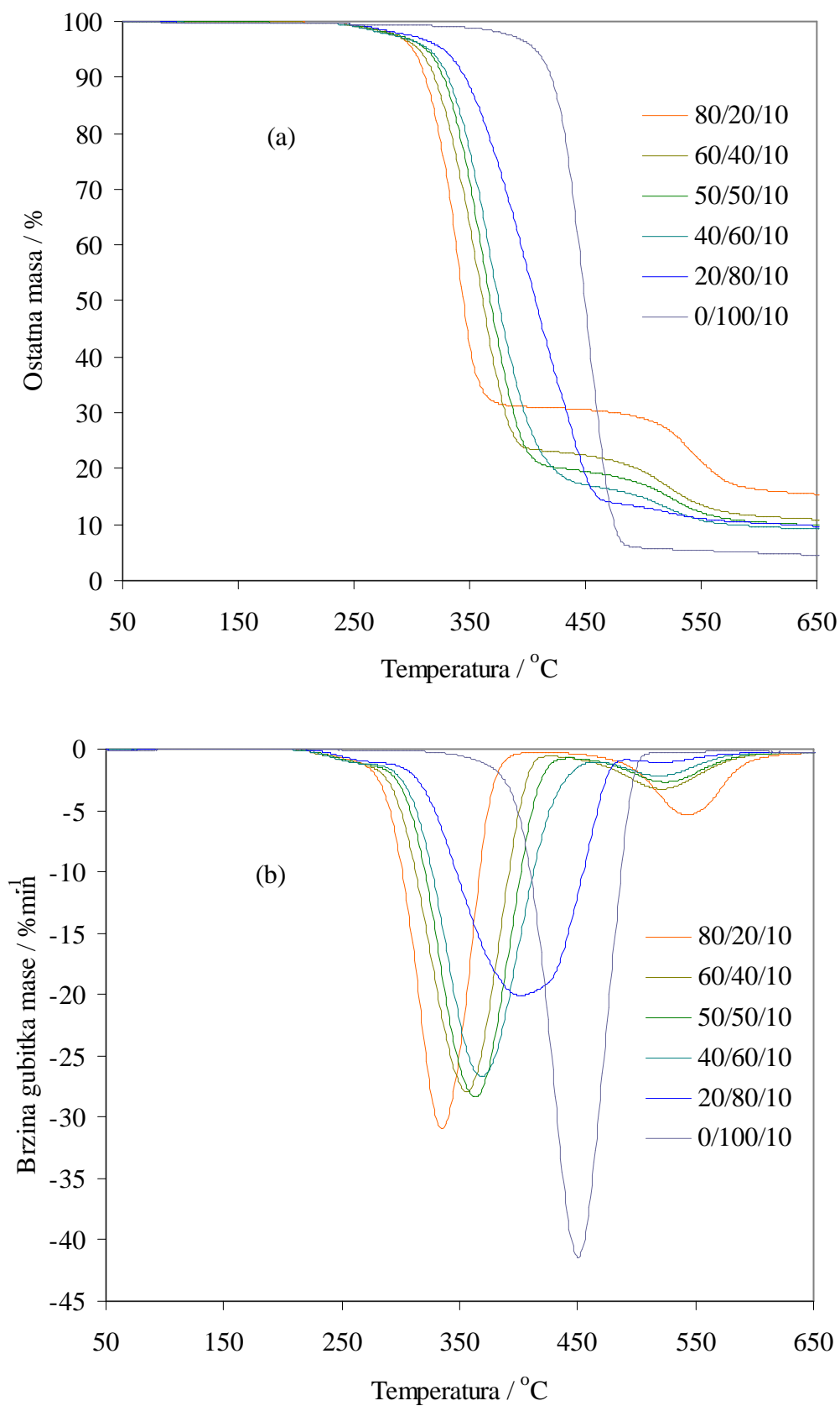
Slika 78. TG (a) i DTG (b) krivulje dinamičke TG razgradnje mješavina PVC/PEO3/PEG različitog sastava u zraku pri brzini zagrijavanja 20\text{ °Cmin}^{-1}
