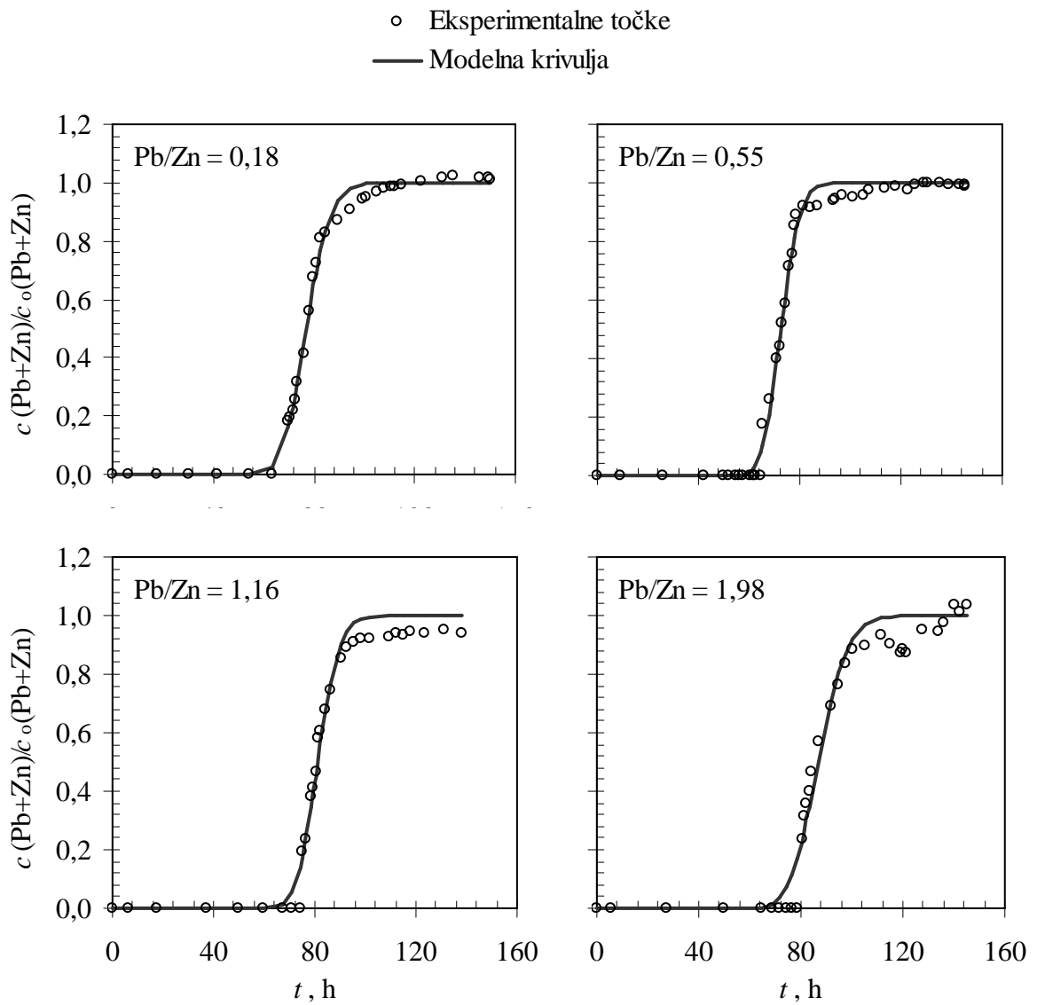
Slika 5.42. Usporedba eksperimentalnih točaka i modelnih krivulja probija prema ADR modelu za visinu sloja zeolita od H = 12 cm i različite Pb/Zn omjere.
