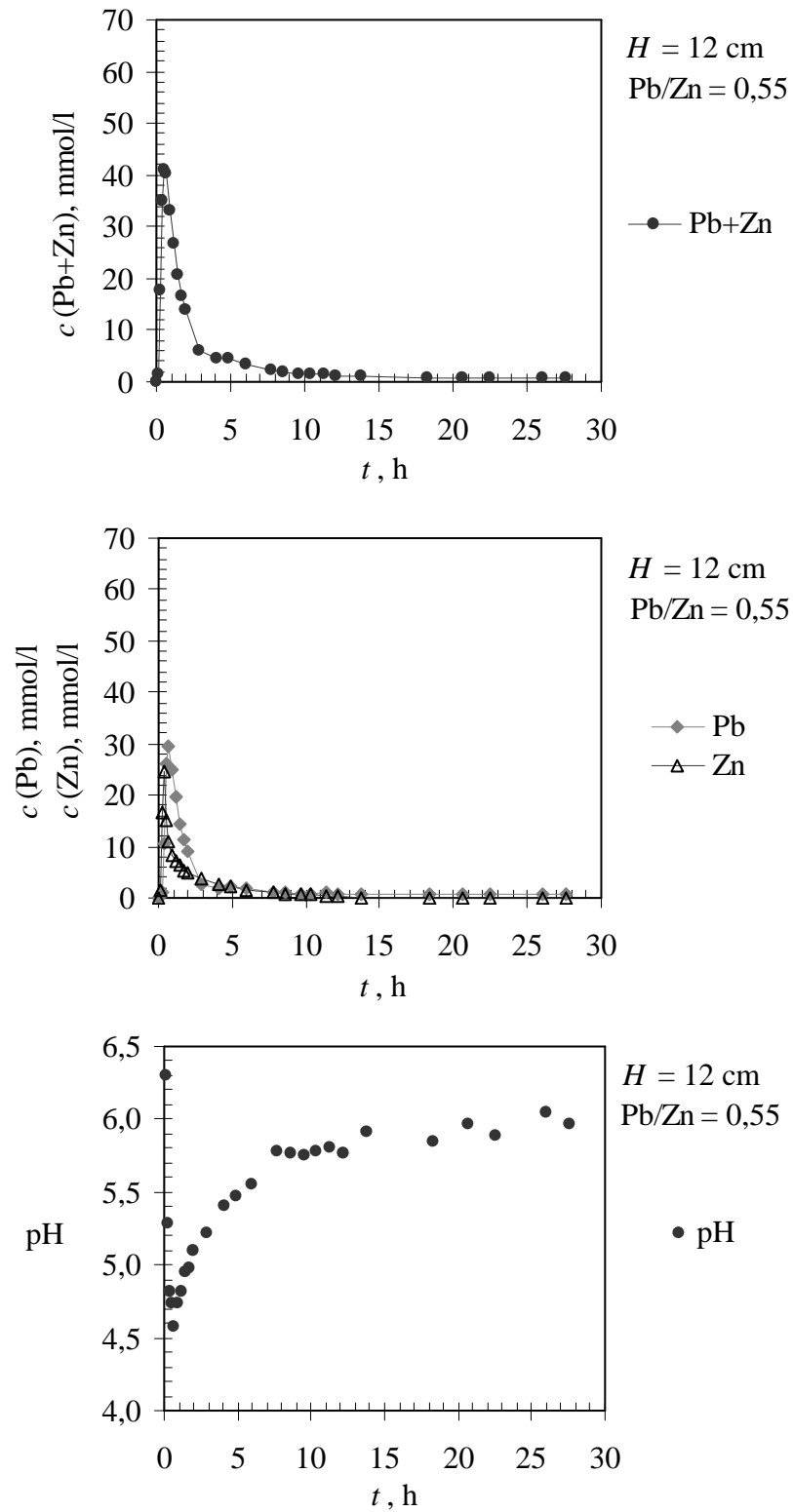
Slika 5.24. Krivulje regeneracije za visinu sloja zeolita H = 12 \text{ cm} i \text{Pb/Zn} = 0,55 za: a) ukupnu koncentraciju ( \text{Pb+Zn} ), b) pojedinačne koncentracije \text{Pb} i \text{Zn} i c) pH vrijednost.
