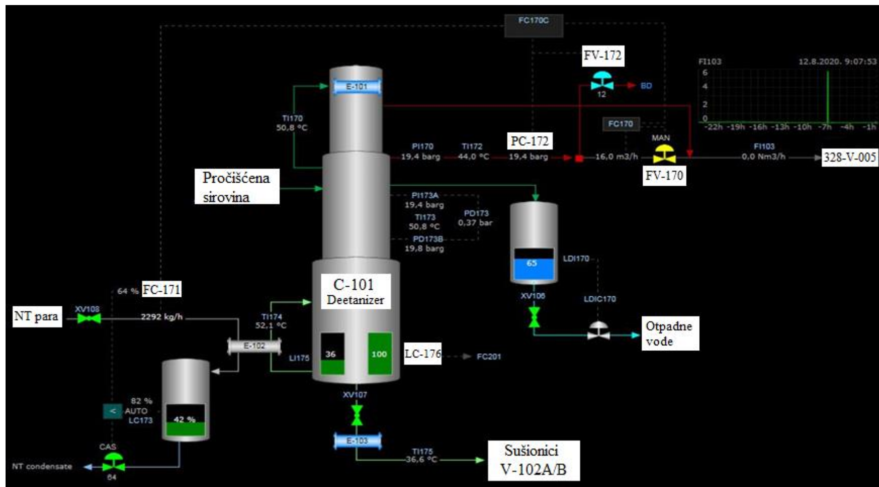
Slika 1.10. Deetanizer kolona. 12
