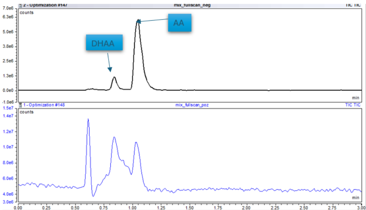
Slika 16. Usporedba pozitivnog i negativnog načina rada kromatografa
