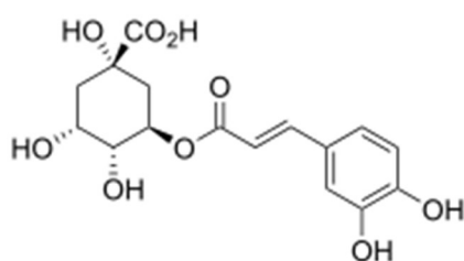
Slika 1. Kemijska struktura klorogenske kiseline 6
