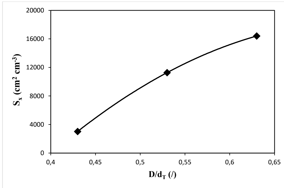
Slika 35. Promjena specifične površine, S_x , finalnog produkta ultrazvučne kristalizacije boraksa s promjerom SBT miješala ( N = N_{JS} ; T_s = 30 °C; b = 6 °C h -1 ; A = 20\% ; p = 20\% ).
