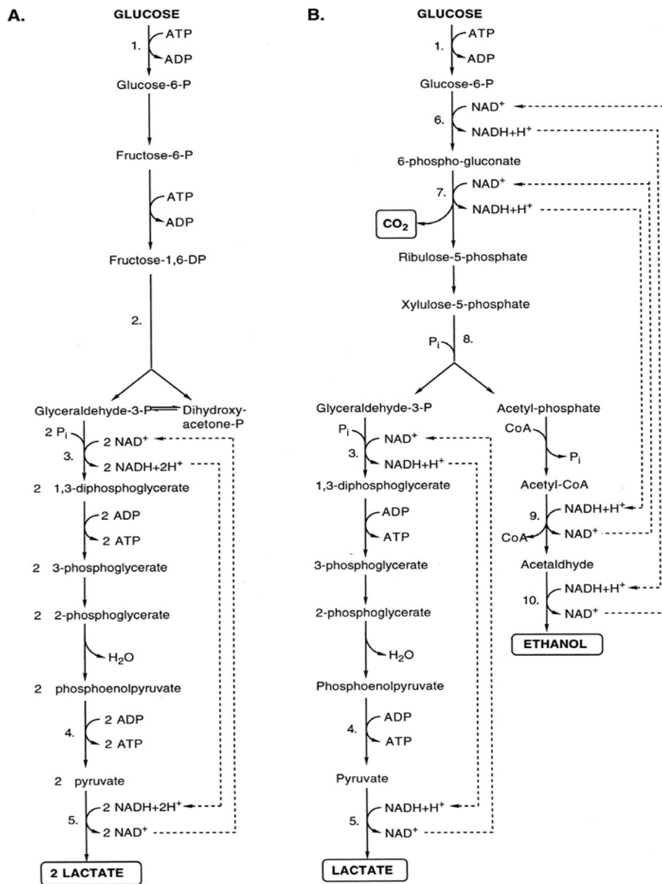
Slika 2. Glavni putevi fermentacije glukoze: (A) homolaktička fermentacija (glikoliza, Embden-Meyerhof-Parnasov put); (B) heterolaktička fermentacija (put 6-fosfogluconata/fosfoketolaze). Enzimi u glavnim putevima fermentacije glukoze: 1. glukokinaza; 2. fruktoza-1,6-difosfat aldolaza; 3. gliceralhid-3-fosfat dehidrogenaza; 4. piruvat kinaza; 5. laktat dehidrogenaza; 6. glukoza-6-fosfat dehidrogenaza; 7. 6-fosfogluconat dehidrogenaza; 8. fosfoketolaza; 9. acetalhid dehidrogenaza; 10. alkohol dehidrogenaza. 20
