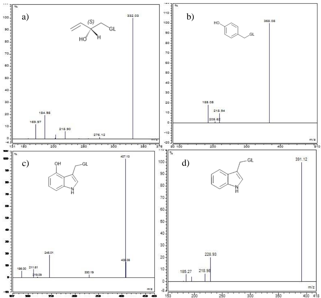
Slika 24. Spektar masa: a) desulfoepiprogoitrin b) desulfofoglukosinalbin c) desulfo4-hidroksiglukobrasicin d) desulfofoglukobrasicin
