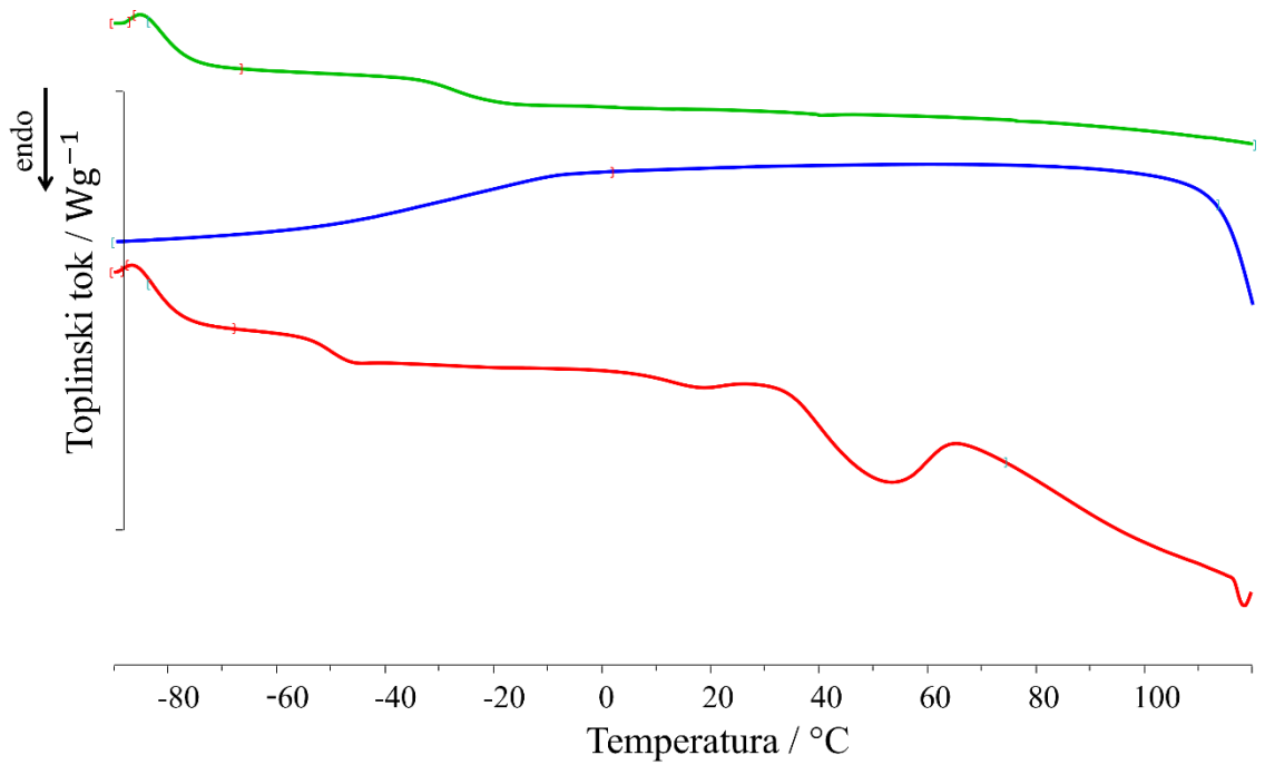
Slika 9. Normalizirane DSC krivulje uzorka PEO/LiMMT/LiBOB 1/7
