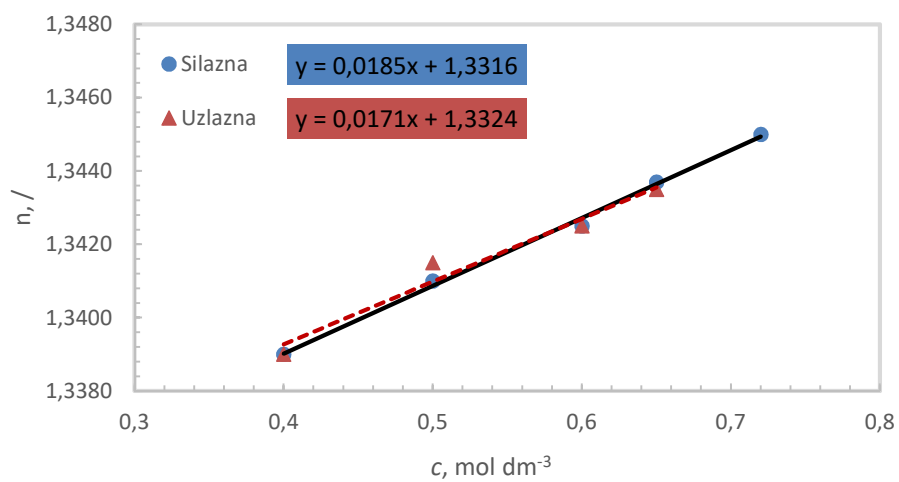
Slika 21. Baždarni pravci za silazno i uzlazno mijenjanje temperature pri T = 35 \text{ °C} .
