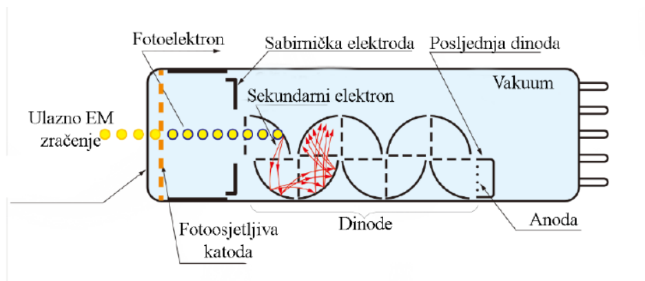
Slika 9. Shematski prikaz fotomultiplikatora 14
