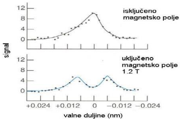
Slika 14. Zeemanov efekt 14
